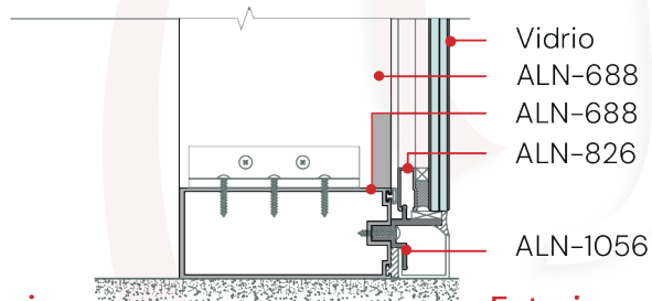
Det. 03
