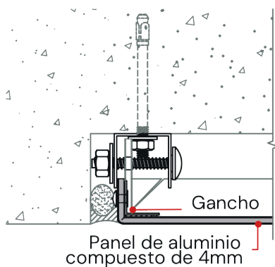
Det. 04
