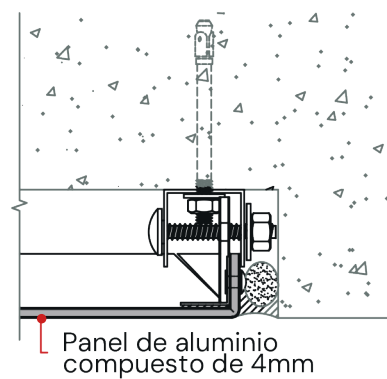
Det. 06
