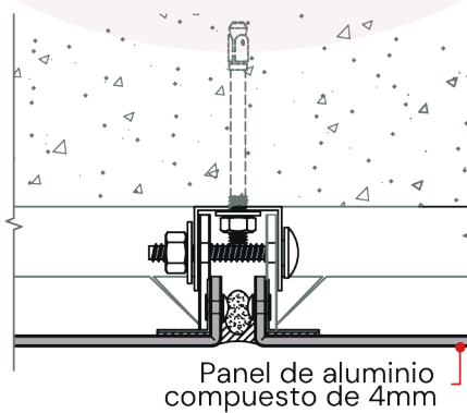
Det. 05
