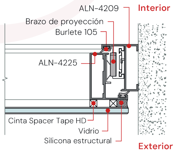
Det. 02
