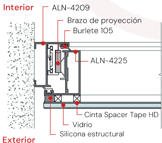
Det. 01
